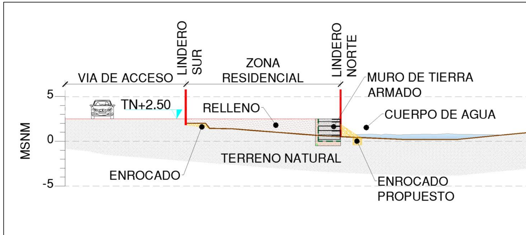
Figura 8 Sección transversal tipo de la solución hidráulica
